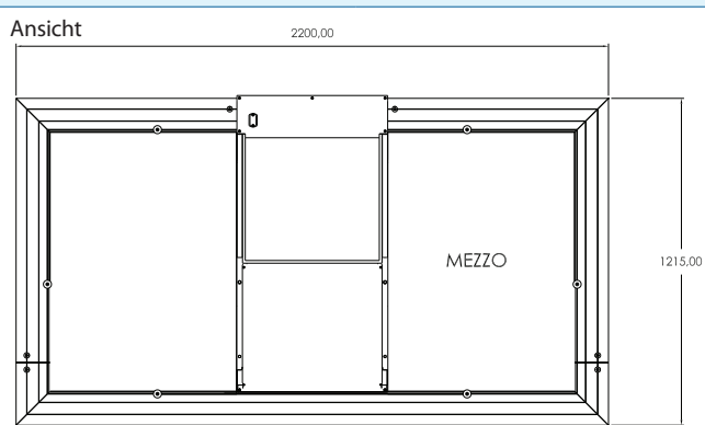
Raucherkabine Mezzo / Mezzo PA
