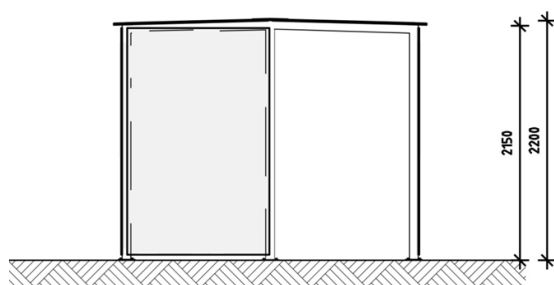
Vorderansicht
