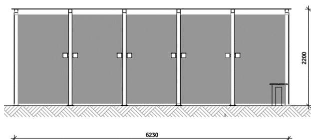
Querschnitt
