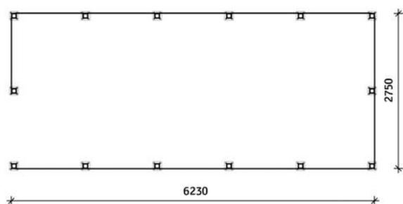
Grundriss
